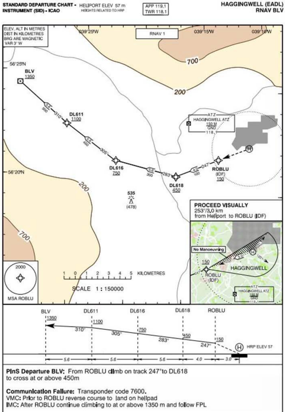
Przykładowa mapa nr 6. Odlot do punktu w przestrzeni (PinS) dla śmigłowców
