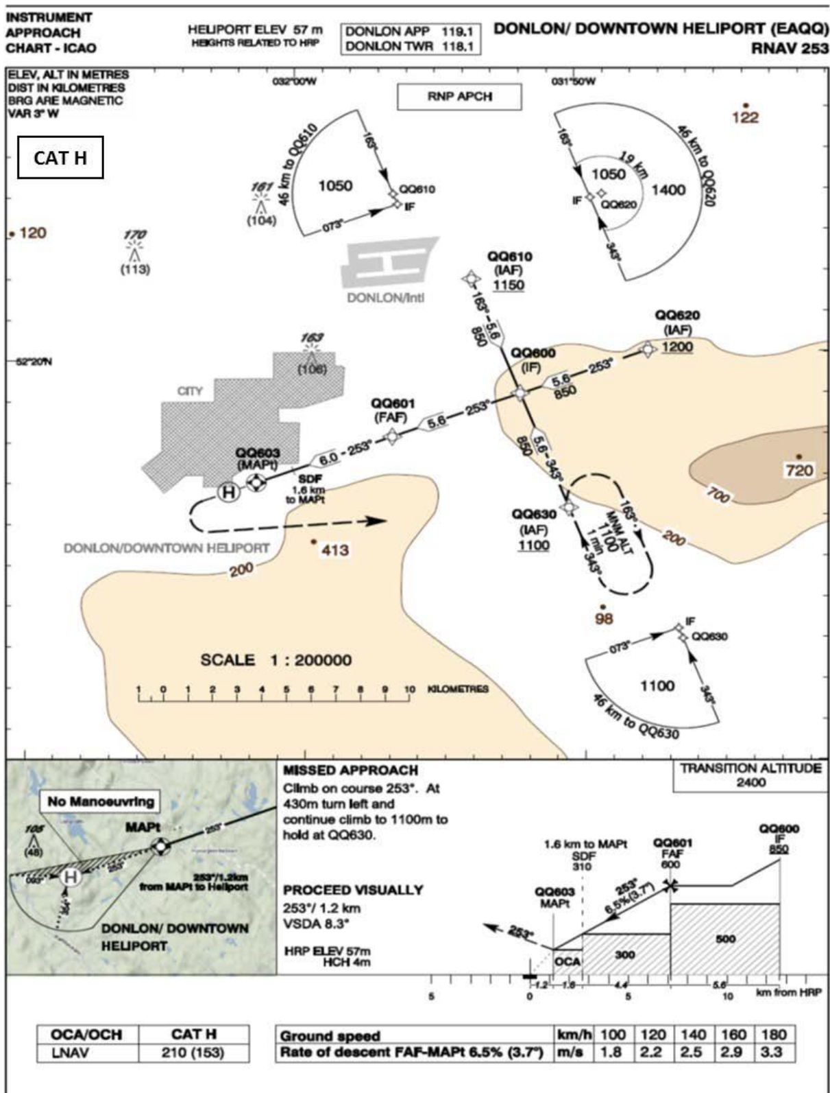
Przykładowa mapa nr 8. Podejście do punktu w przestrzeni dla śmigłowców do minimów LNAV (lot z widocznością)
