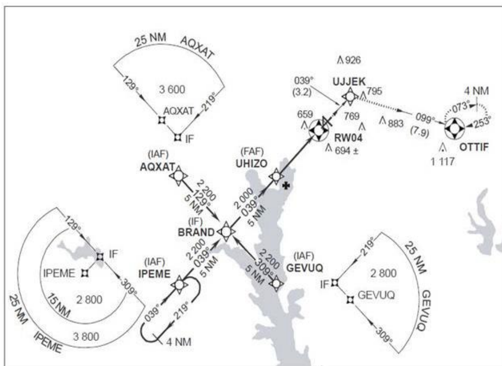
Rysunek 6.1. Obszar dołotu w rejon lotniska
