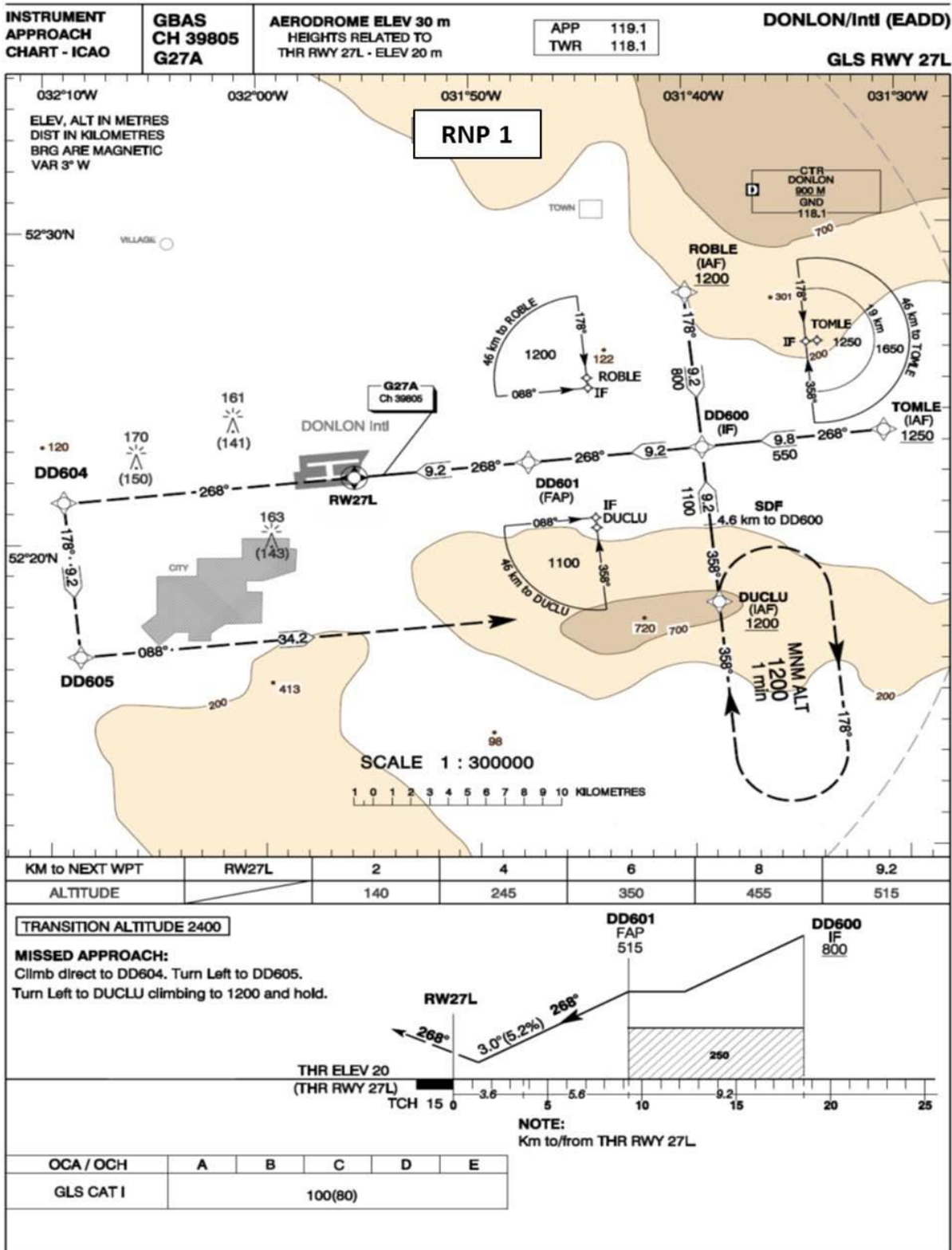
Przykładowa mapa nr 4. Podejście GLS z segmentami PBN
