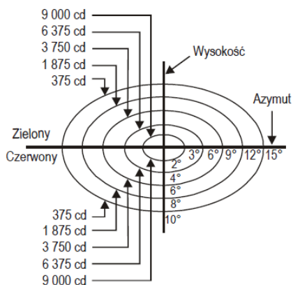
Ilustracja 4 – System HAPI
