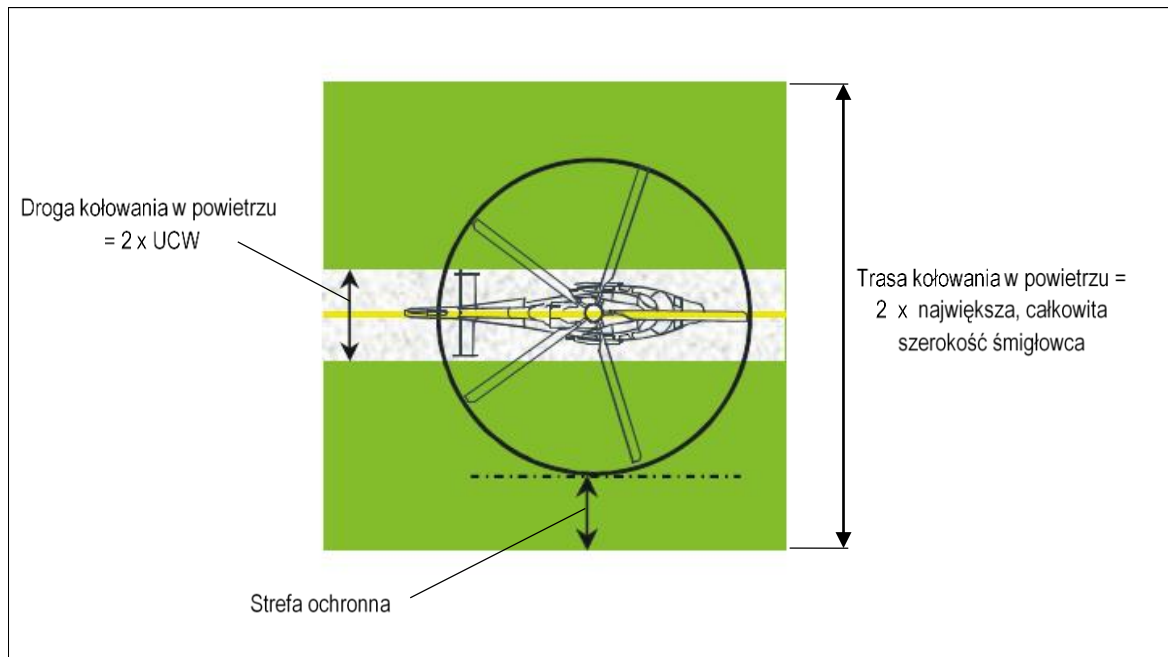
Rysunek 3-3. Droga kołowania / trasa kołowania śmigłowców w powietrzu
