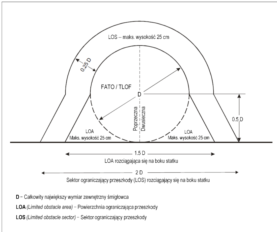
Rysunek 4.11. Sektory i powierzchnie ograniczające przeszkody na prowizorycznym lotnisku dla śmigłowców zlokalizowanym w bocznej części statku
